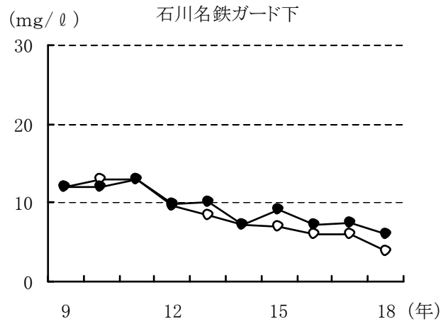
図2. 2 河川BOD・COD経年変化
