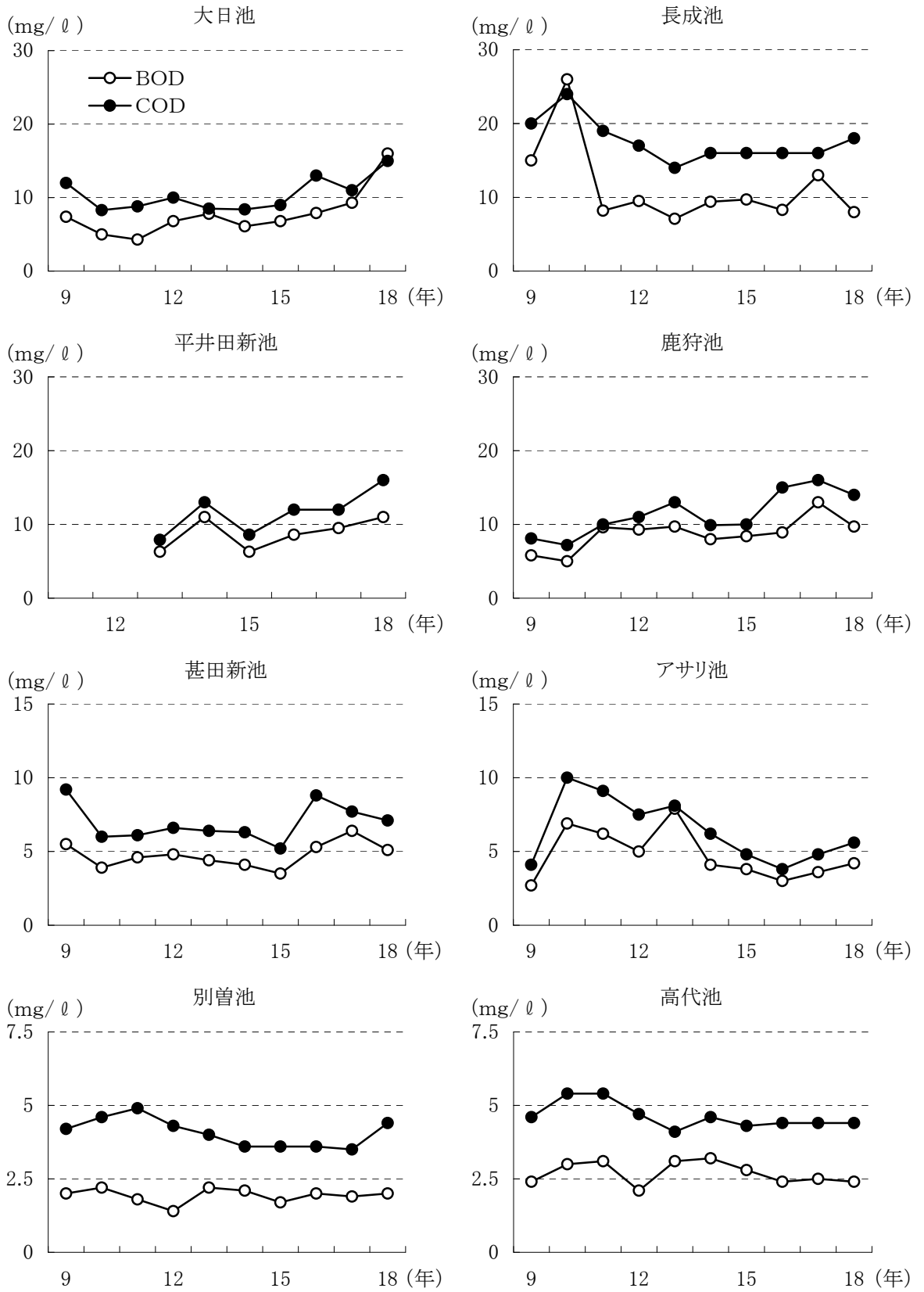
図2.3 ため池BOD・COD経年変化
