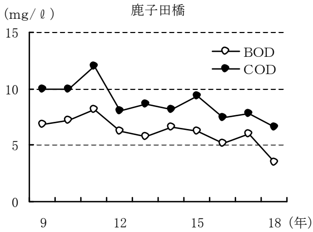
図2. 2 河川BOD・COD経年変化
