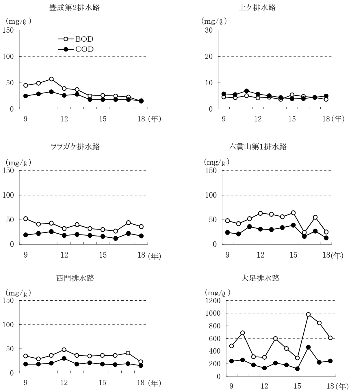
図2. 4 排水路BOD・COD経年変化
