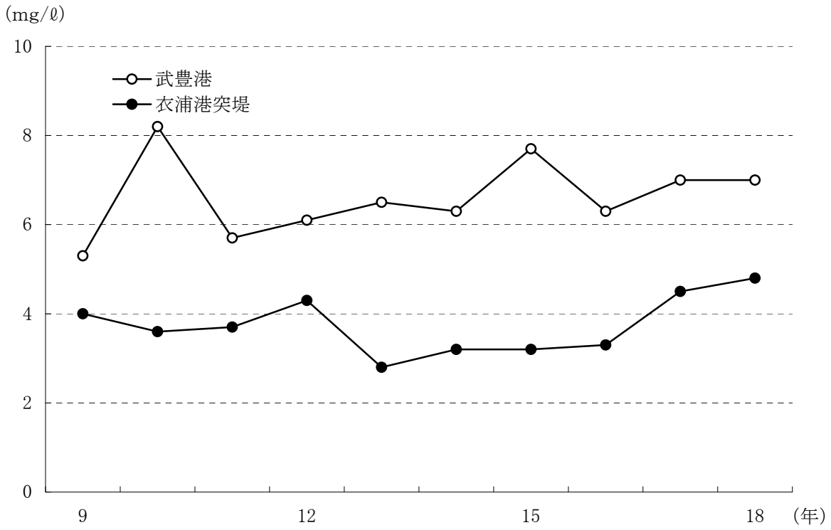
図2.6 海水COD経年変化
