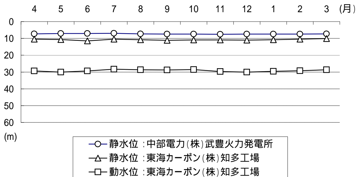
図5.2 地下水位経月変化
