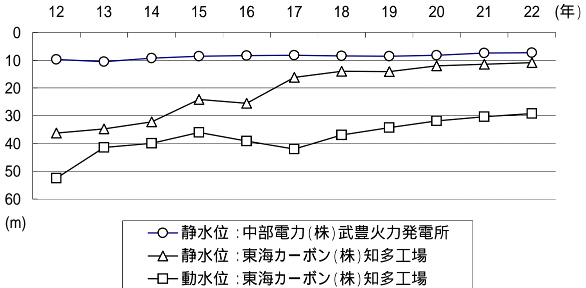
図5.1 地下水位経年変化
