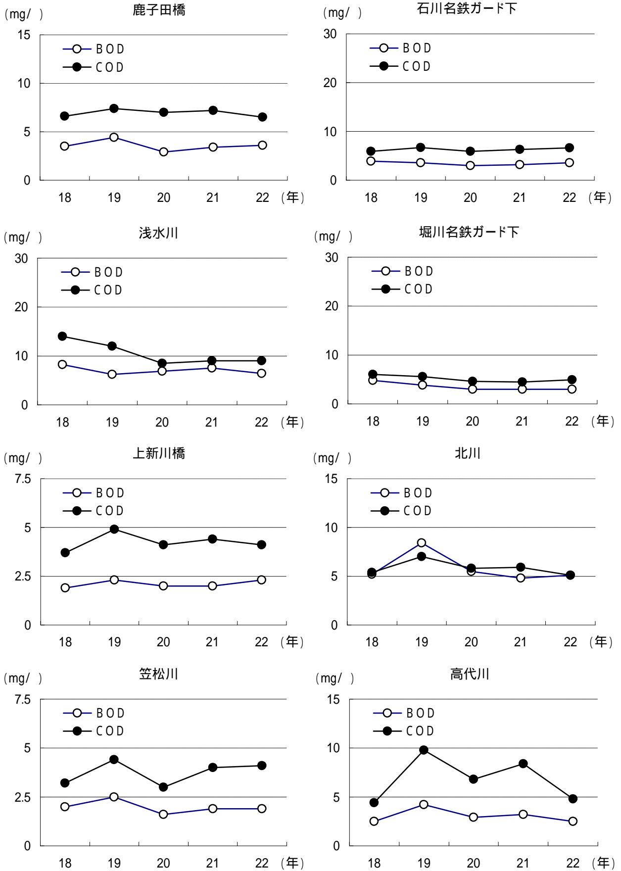
図 2 . 2 河川 B O D ・ C O D 経年変化
