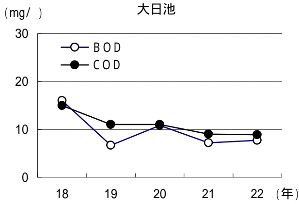
図 2 . 3 ため池 B O D ・ C O D 経年変化
