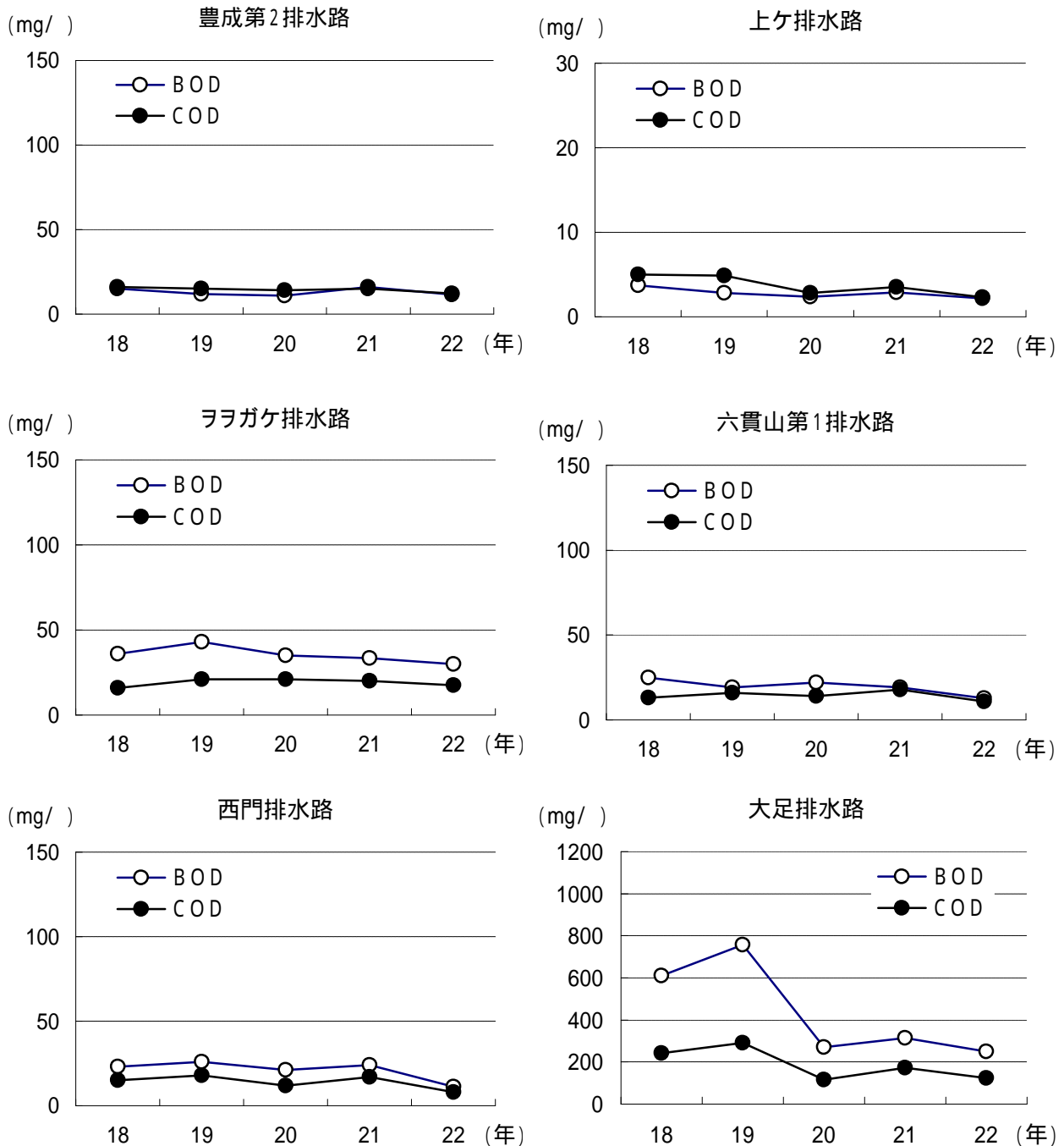
図 2.4 排水路BOD・COD経年変化
