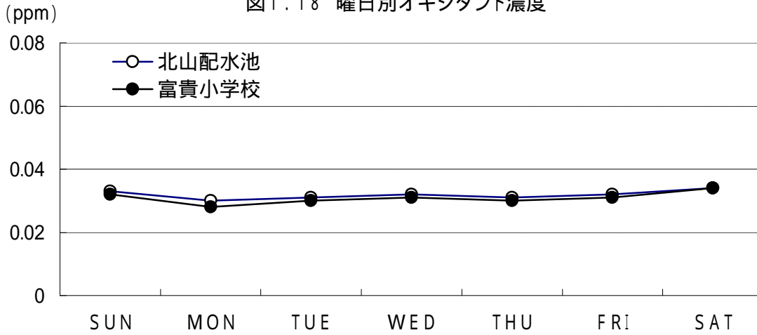
図1.18 曜日別オキシダント濃度
