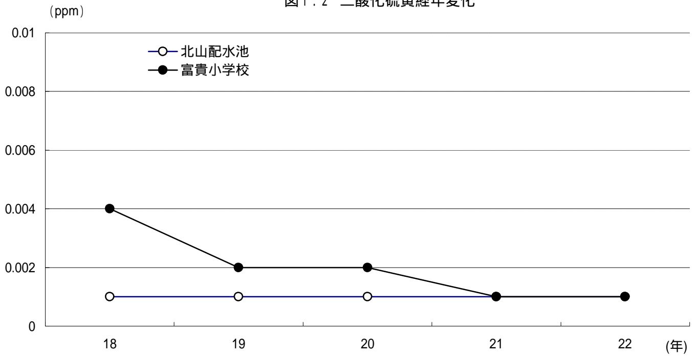
图1.2 二酸化硫黄経年变化
