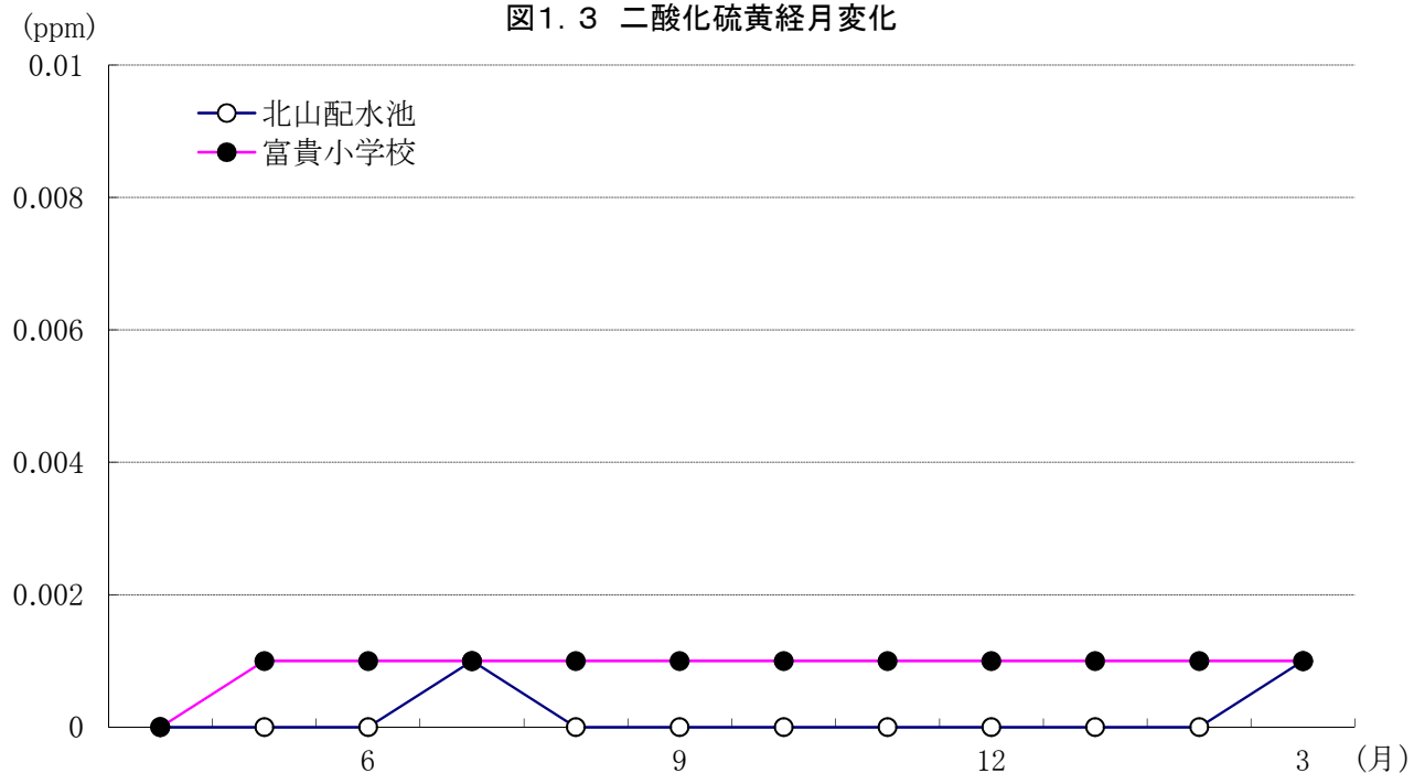
图1.3 二酸化硫黄経月変化
