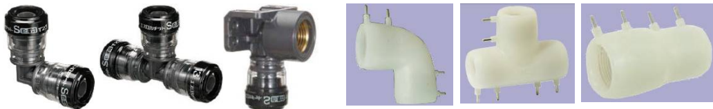
図4-1 ポリエチレン・ポリブデン管の継手類 [クイック式]・[電気融着式]
