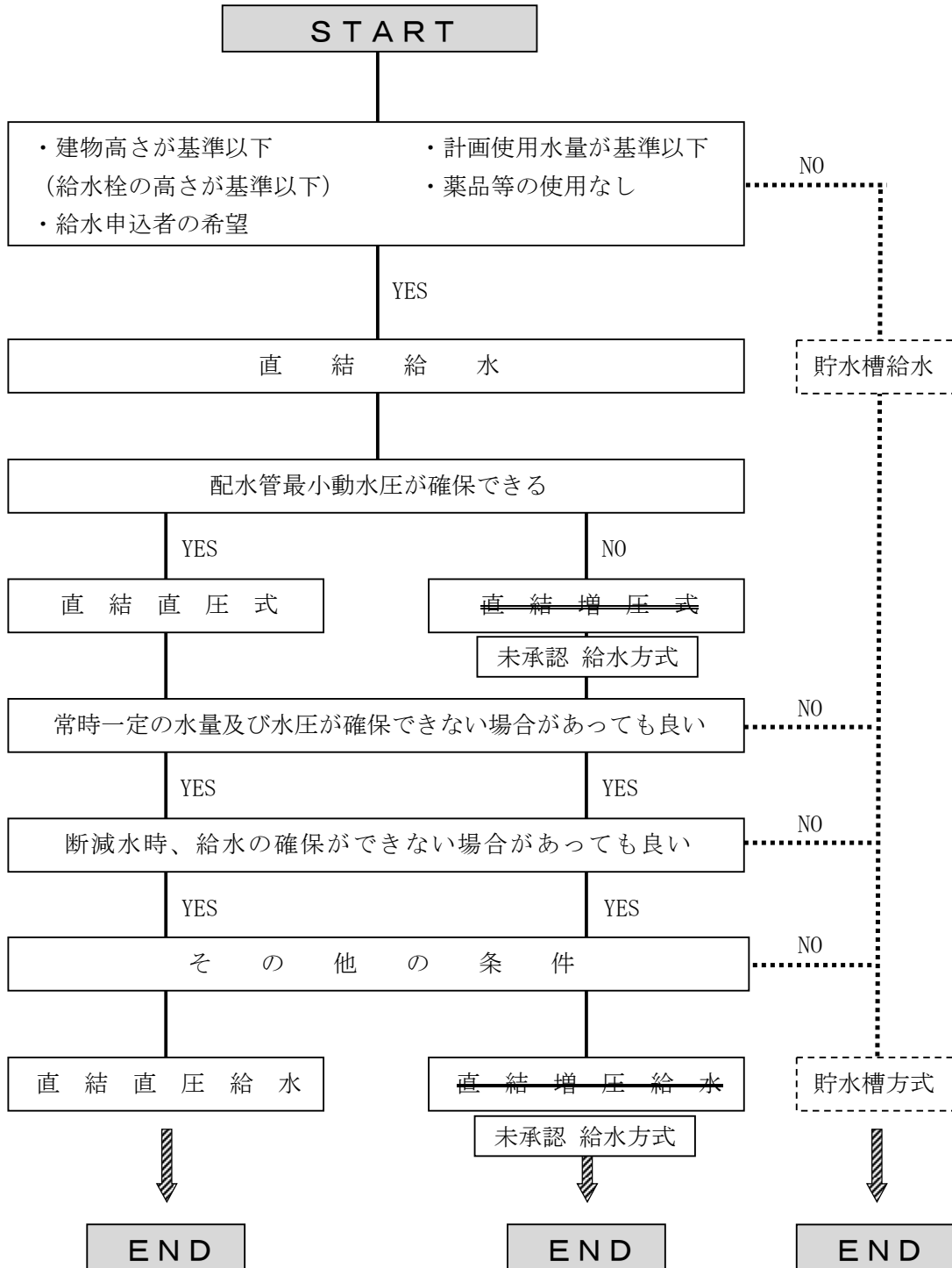
図1-2 給水形態の選定フロー (例)
