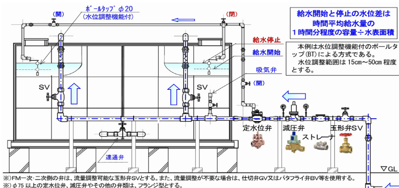
図6-8 受水槽周り(一弁二槽型)の配管要領図
