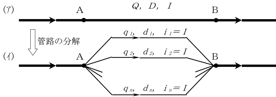
図 3-12 管路の平行閉管路への分解図 ( (a) ⇒ (b) )
