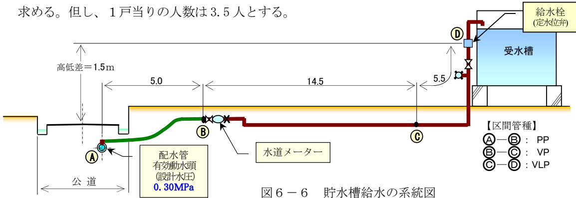
図6-6 貯水槽給水の系統図
