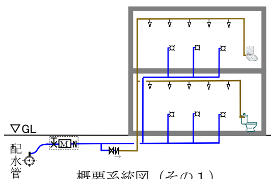
概要系統図 (その 1)
