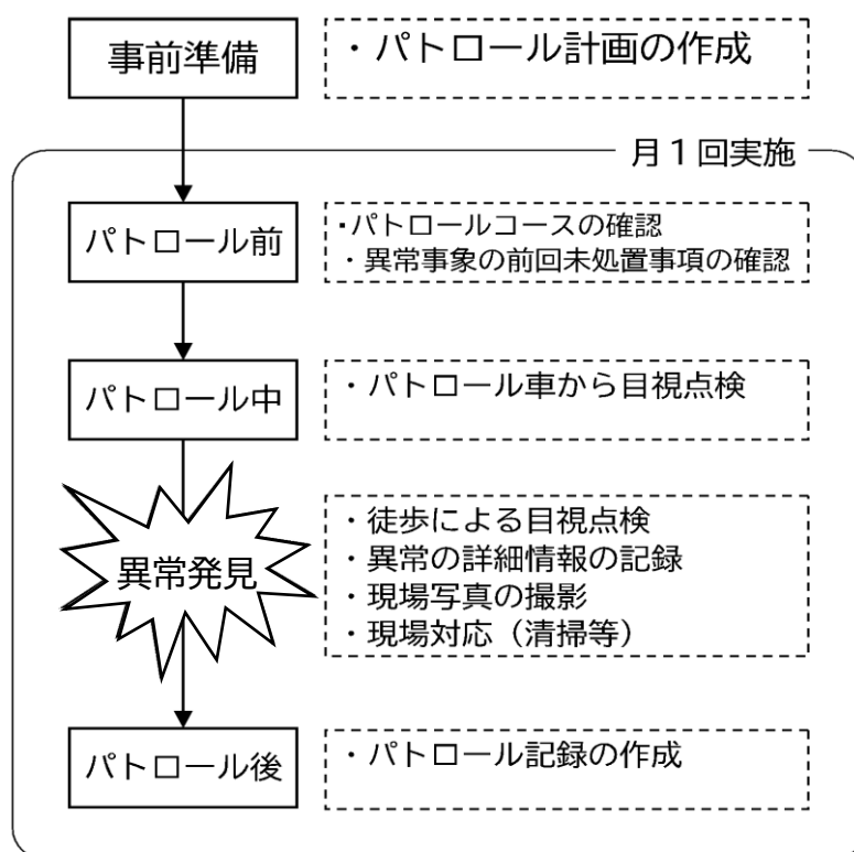
道路パトロール実施フロー
