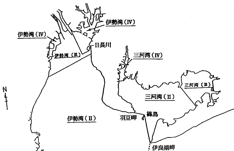
図2.5 伊勢湾・三河湾における全窒素及び全りに係る環境基準の水域類型指定
