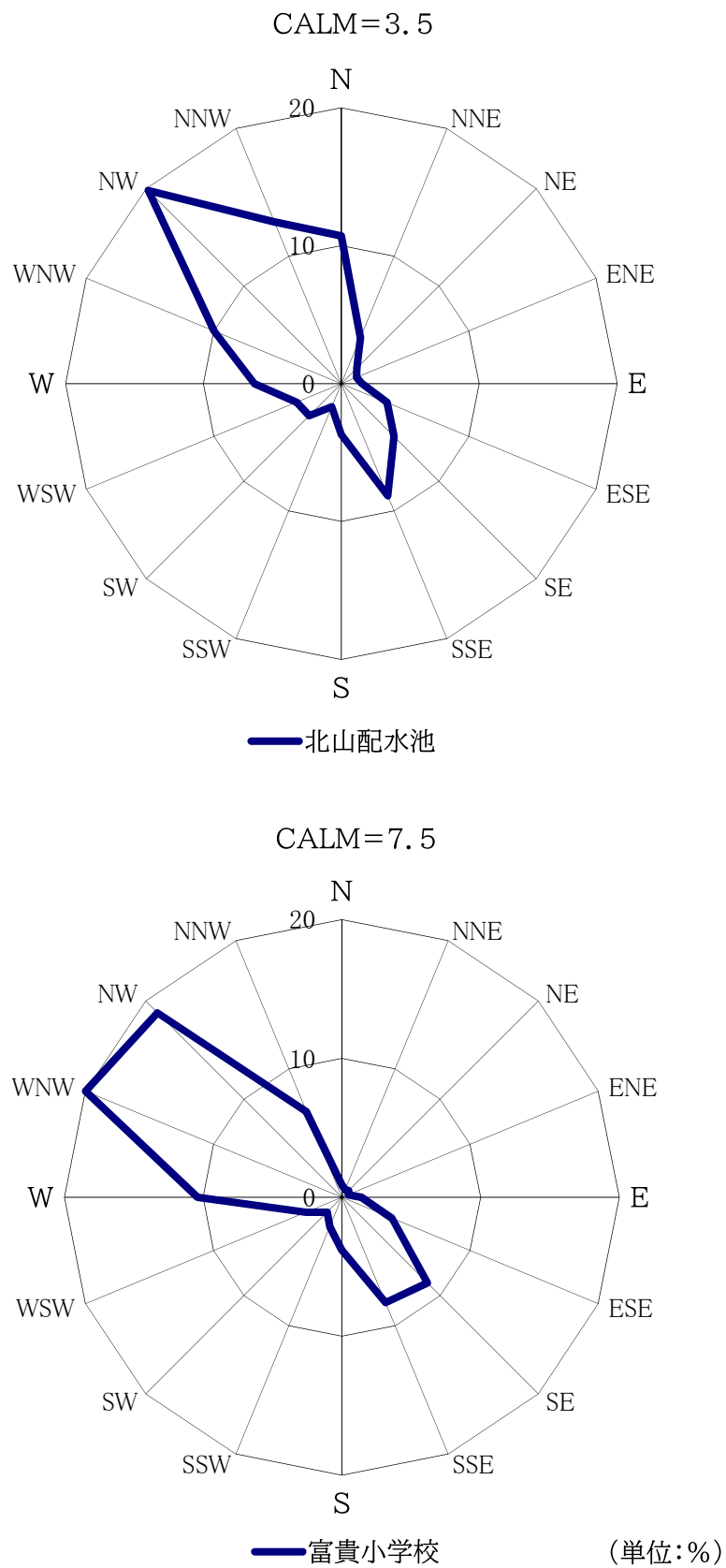
図1. 28 風配図(年間)
