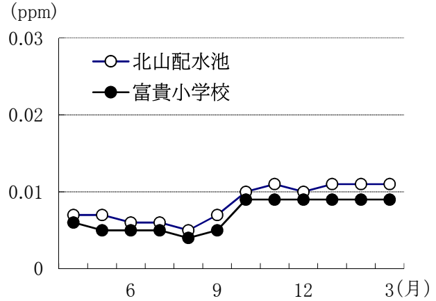
图1.10 二酸化窒素経月变化
