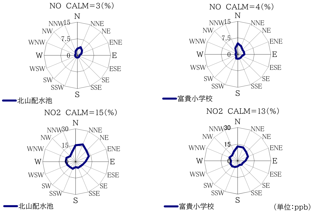
图1.11 風向別窒素氧化物濃度
