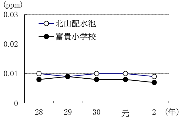
图1.8 二酸化窒素経年变化
