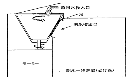
図 スノーボール方式の削氷機械略図(一例) (密閉式の構造を有すること)
